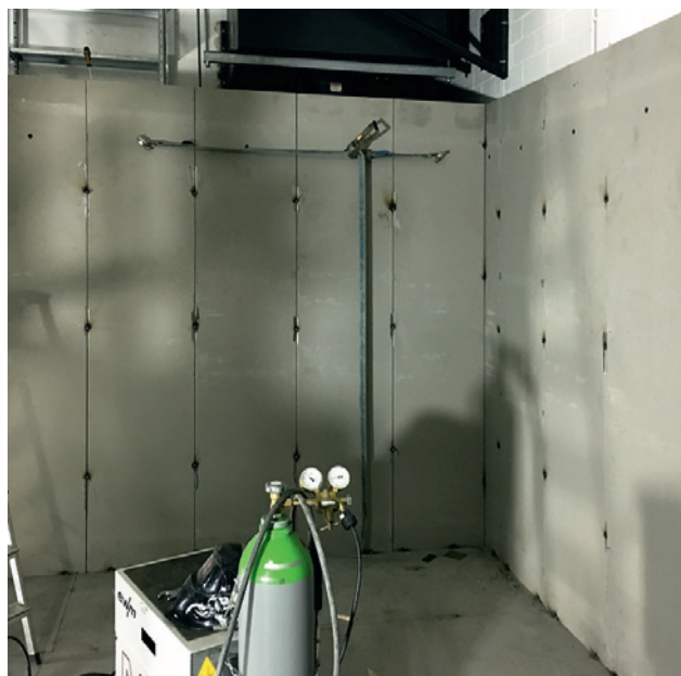
Aufbau Wandelemente (Verschweißung)
